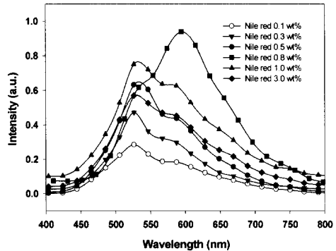
그림 5. ITO/blend(PDPMA-nile red)/Alq 3 /Al 소자의 전기발광 스펙트럼들. Fig. 5. EL spectra of ITO/blend(PDPMA-nile red)/Alq 3 /Al.
