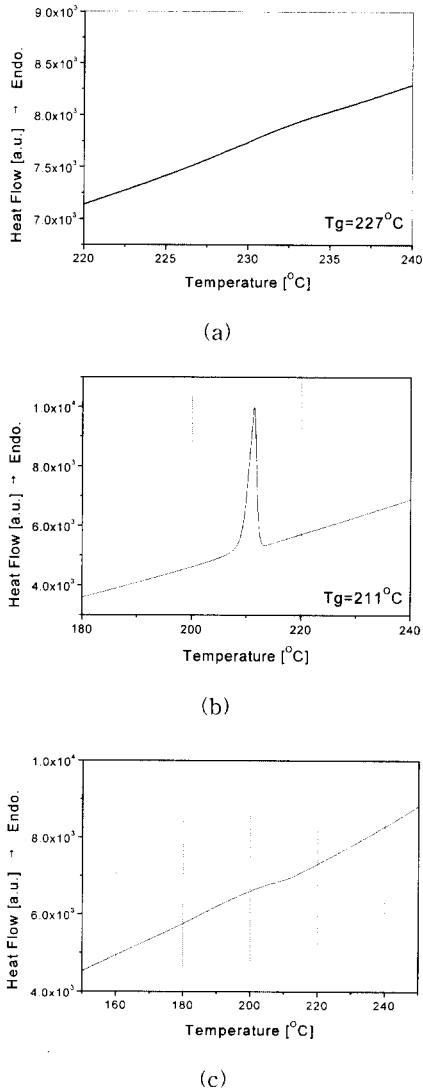
그림 2. DSC 결과.
